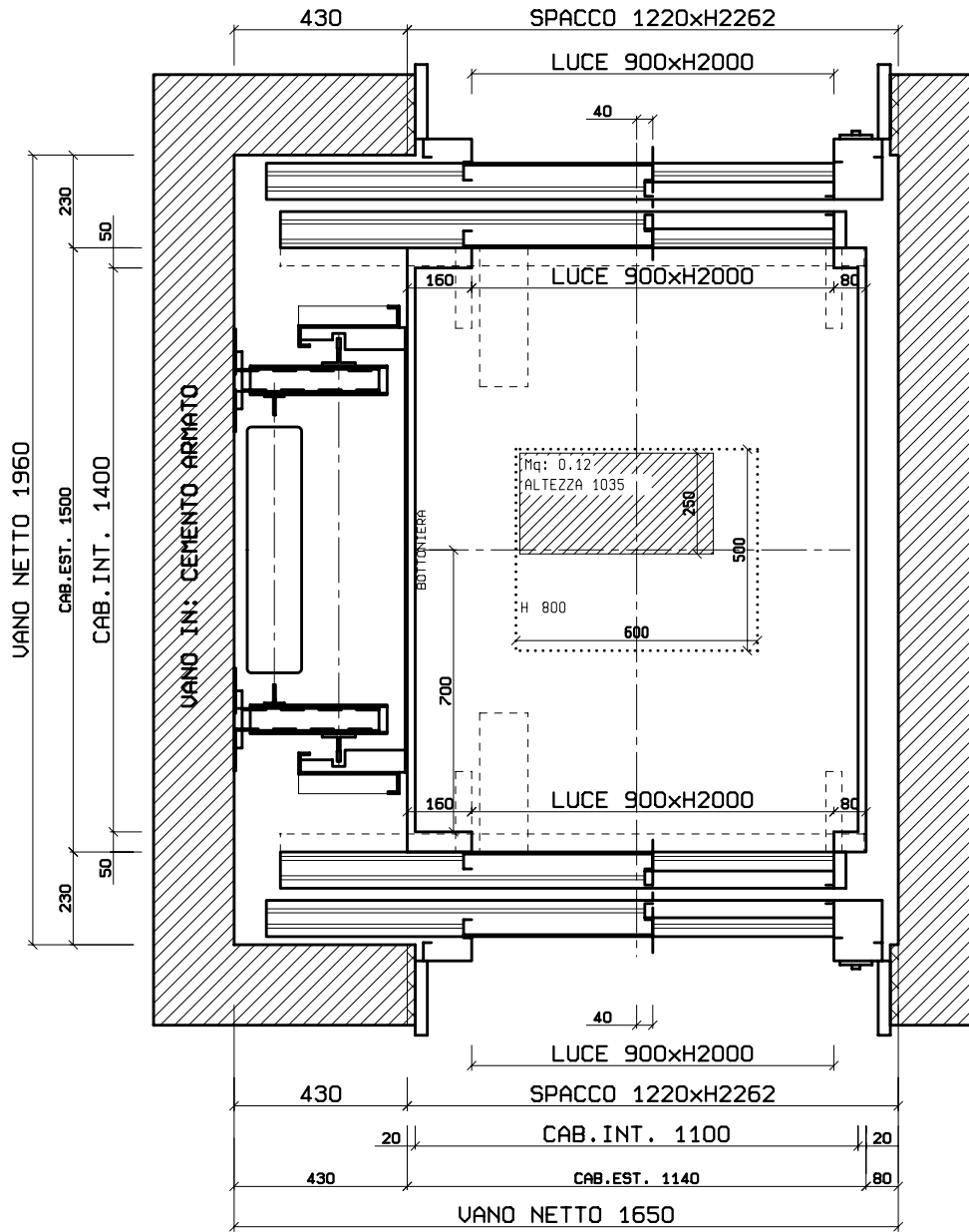
PIANTA VANO CORSA ALL'ULTIMO PIANO SERVITO Scala 1:20
