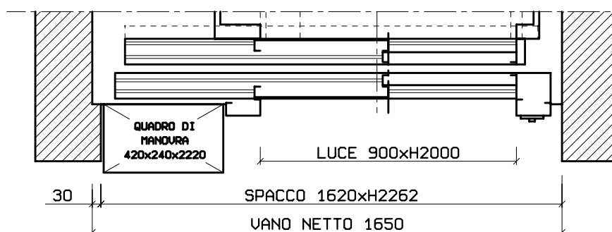
PIANTA VANO CORSA ALL'ULTIMO PIANO SERVITO Scala 1:20
