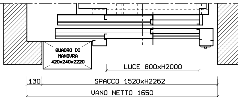
PIANTA VANO CORSA ALL'ULTIMO PIANO SERVITO Scala 1:20
