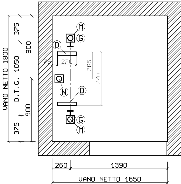
POSIZIONE DEI GANCI DI SOLLEVAMENTO IN TESTATA Scala 1/30
