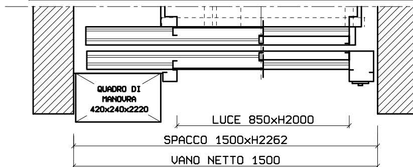
PIANTA VANO CORSA ALL'ULTIMO PIANO SERVITO Scala 1:20
