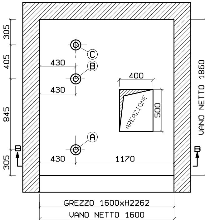
POSIZIONE DEI GANCI DI SOLLEVAZIONE IN TESTATA Scala 1/30
