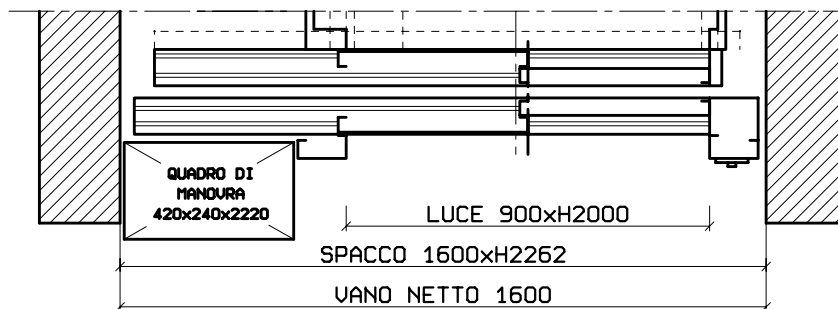
PIANTA VANO CORSA ALL'ULTIMO PIANO SERVITO Scala 1:20
