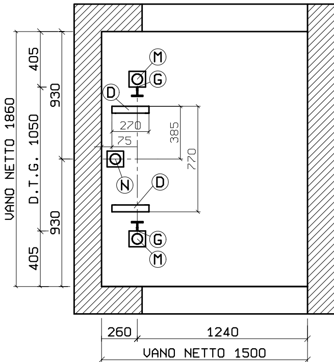
POSIZIONE DEI GANCI DI SOLLEVAZIONE IN TESTATA Scala 1/30
