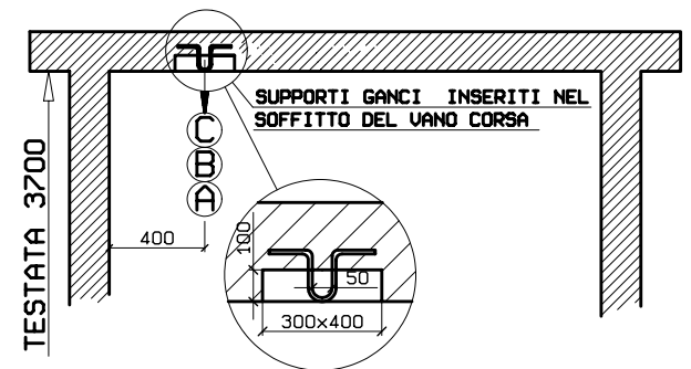
SEZIONE B-B IN TESTATA
