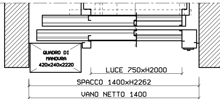
PIANTA VANO CORSA ALL'ULTIMO PIANO SERVITO Scala 1:20
