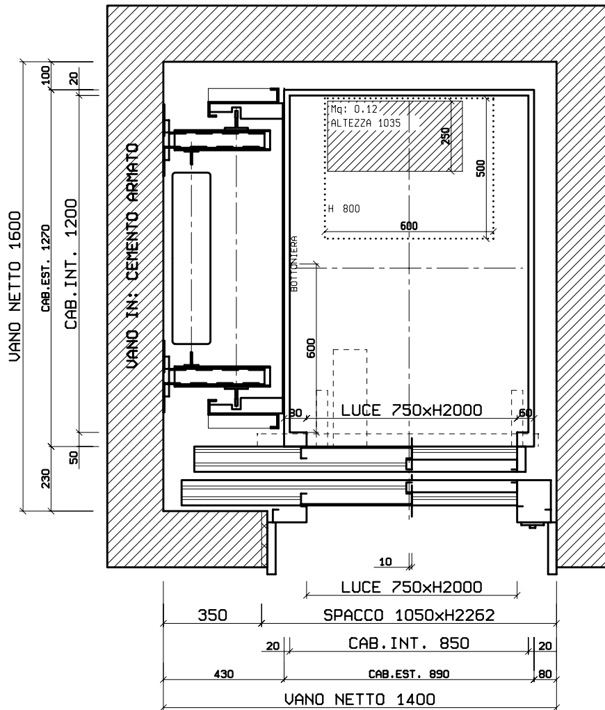
PIANTA VANO CORSA ALL'ULTIMO PIANO SERVITO Scala 1:20
